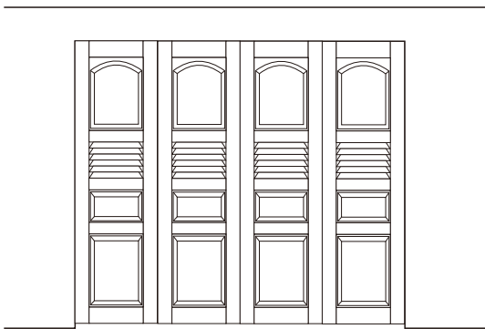
Ilustrasi 4 pintu tampak depan
